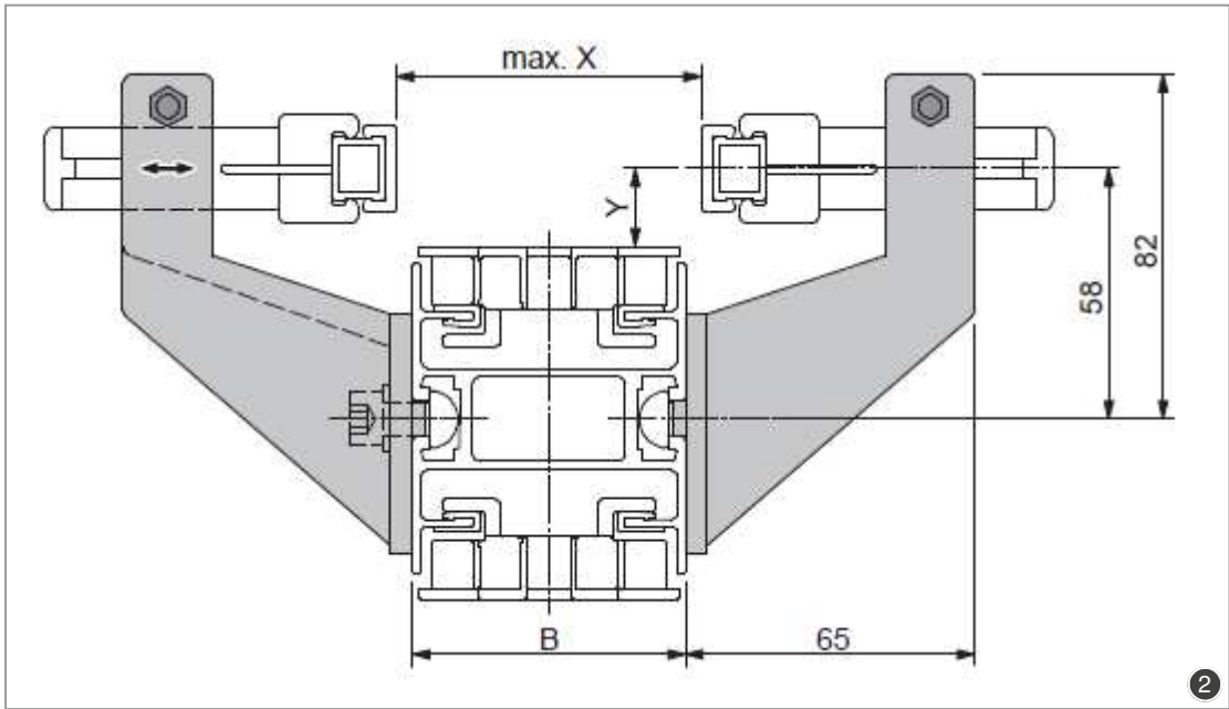
Zijgeleiding steun type 2 • Lateral holder type 2 • Seitenhalter Typ 2
