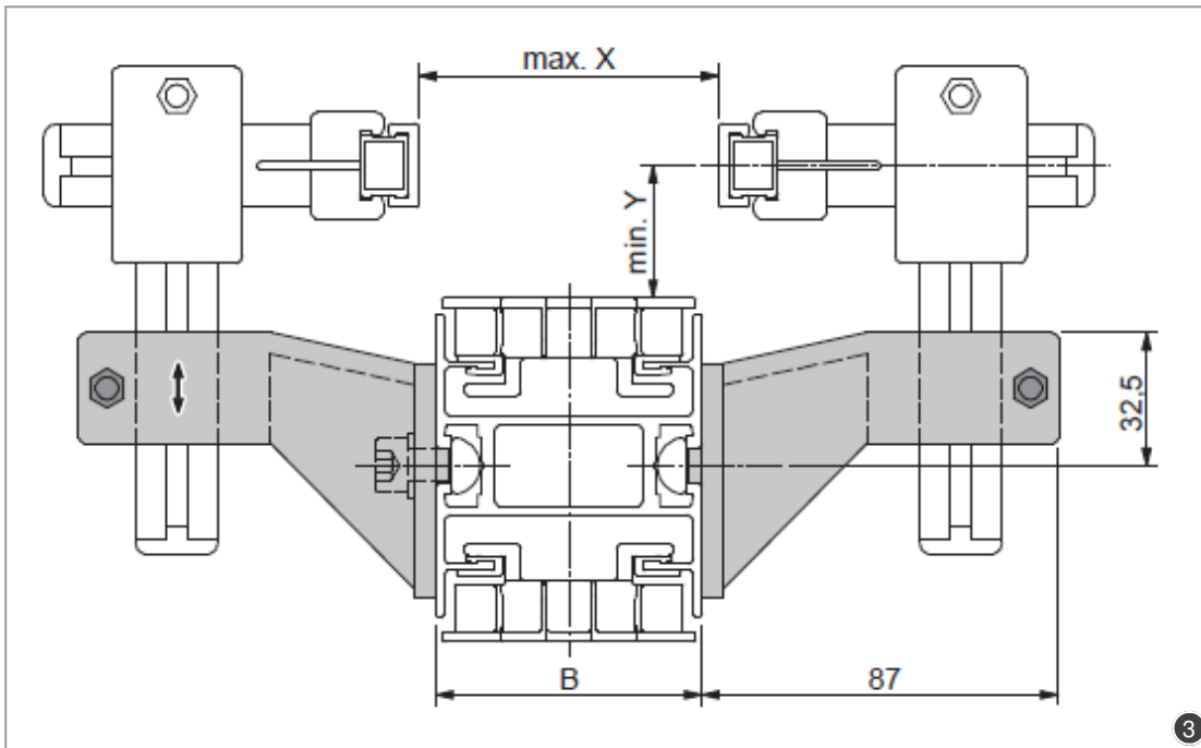
Zijgeleiding steun type 3 • Lateral holder type 3 • Seitenhalter Typ 3
