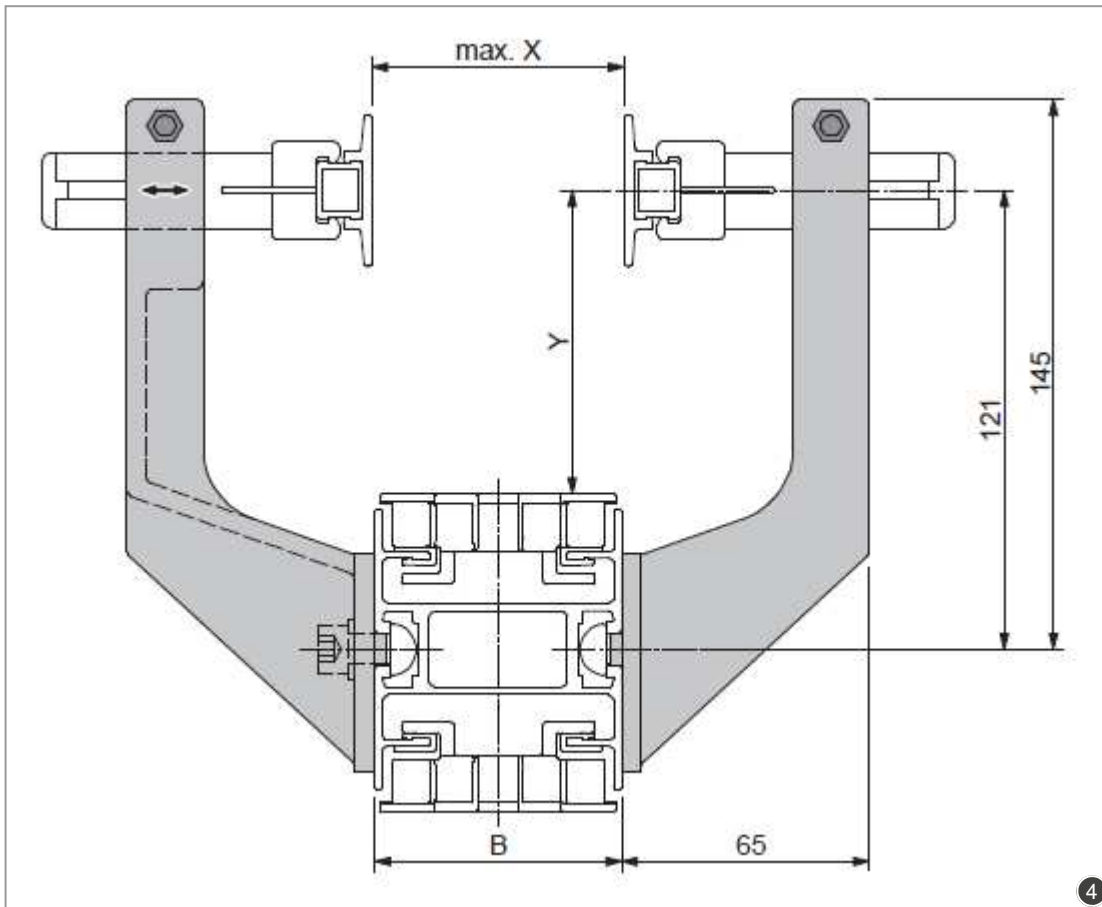
Zijgeleiding steun type 3 • Lateral holder type 3 • Seitenhalter Typ 3
