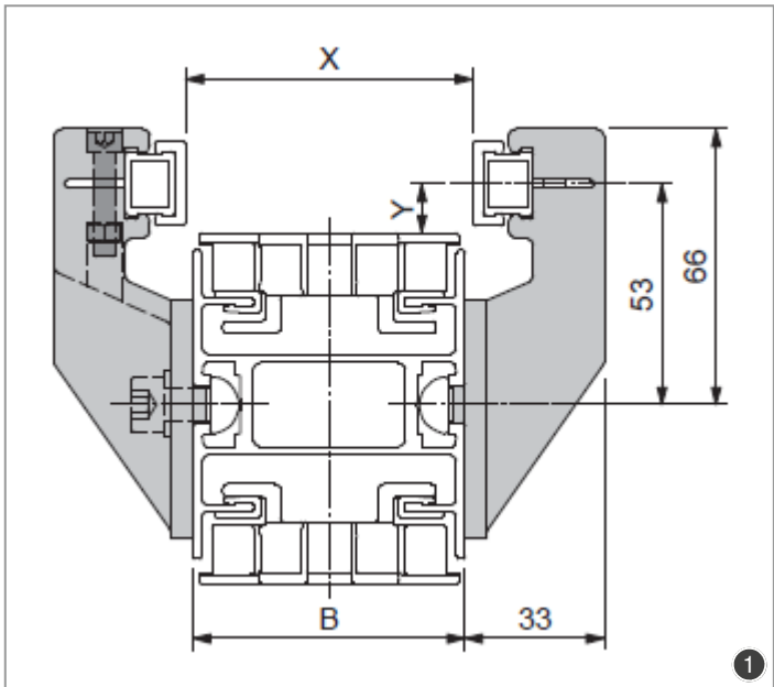
Zijgeleiding steun type 1 • Lateral holder type 1 • Seitenhalter Typ 1
